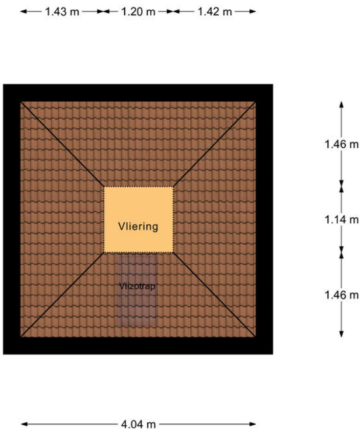
Vliering
